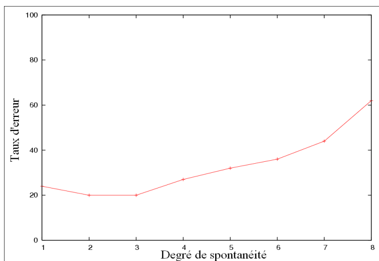
Figure 2. Taux d'erreur de LIUM RT en fonction de la qualité d'élocution
